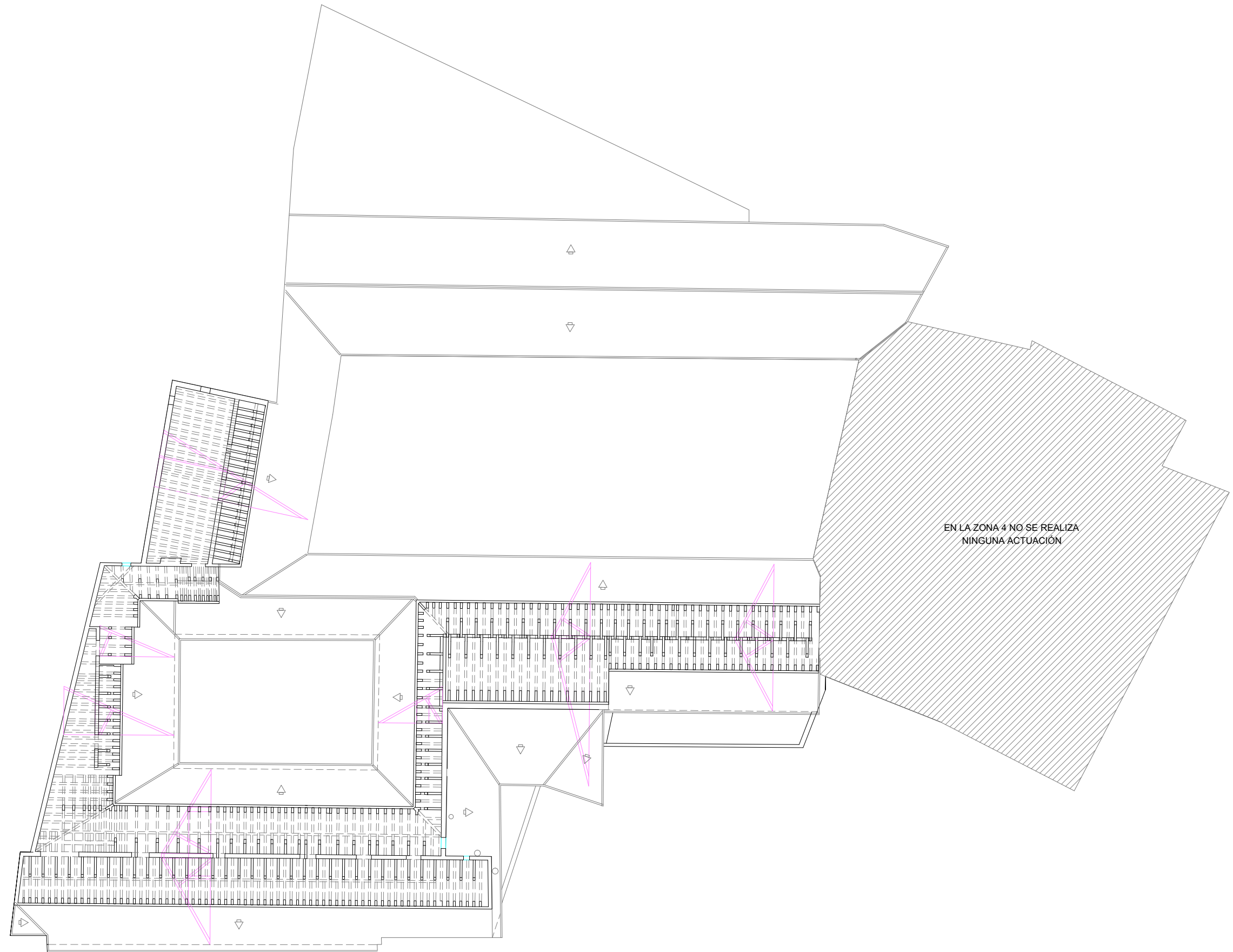
PLANTA BAJO-CUBIERTAS
